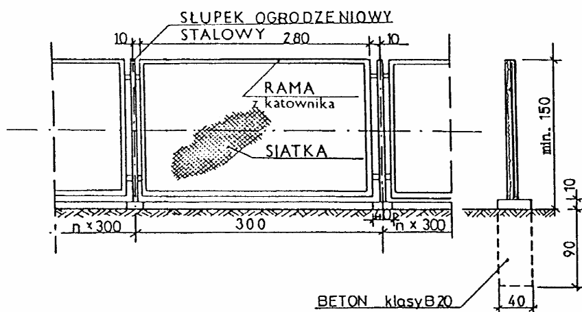
11.1.4. Ogrodzenie z siatki plecione ślimakowej w ramach stalowych z kątownika (wg KPED [44])
