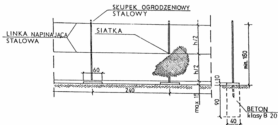
11.1.3. Ogrodzenie z siatki plecione ślimakowej na linkach stalowych (wg KPED [44])
